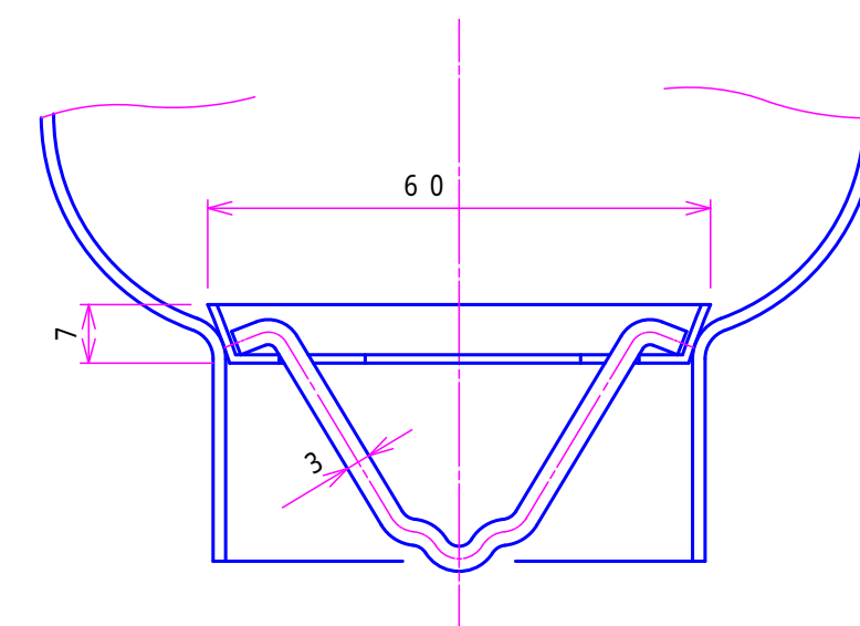
フック詳細
